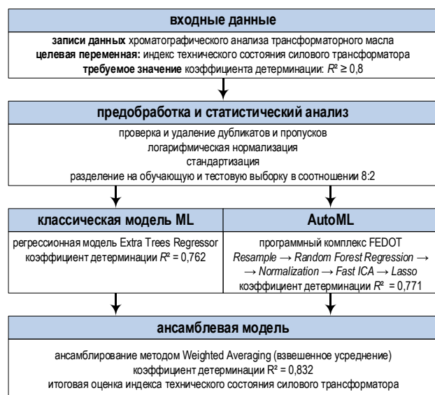
Рис. 5. Структура ансамблевой модели комплексной оценки ТС трансформатора
