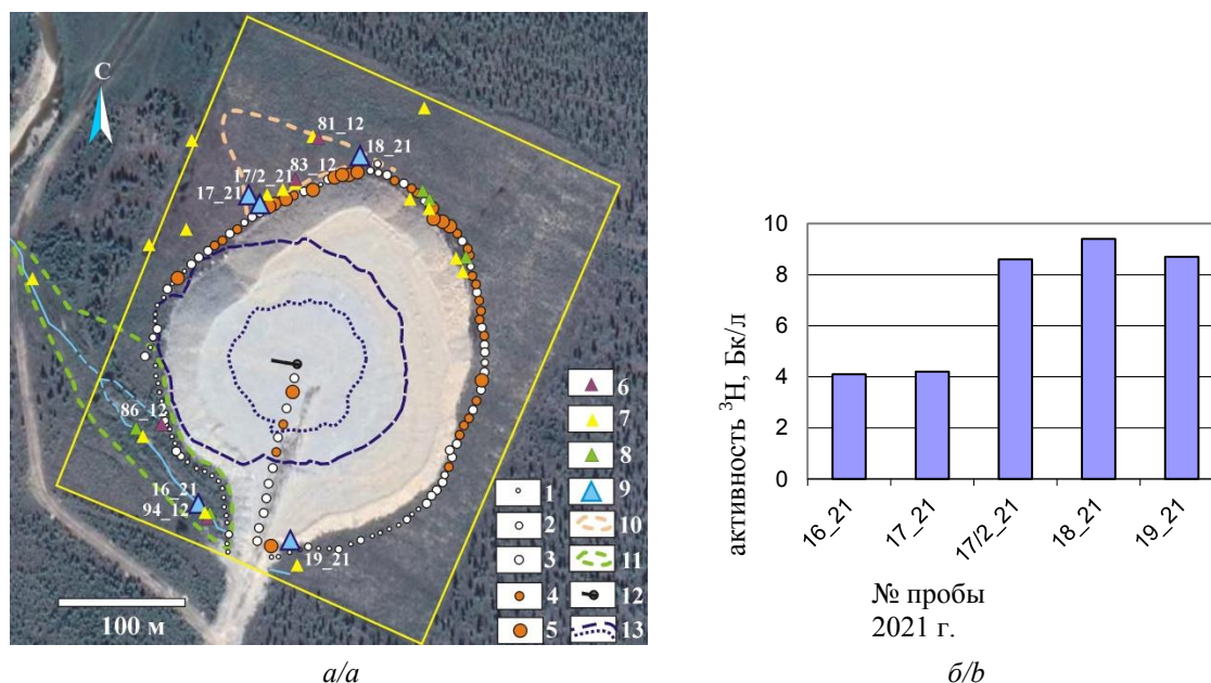
Рис. 3. а) распределение МЭД (мкР/ч): (1) 6–7; (2) 7,5; (3) 8; (4) 8,5; (5) 9–10 в 2021 г. и схема отбора проб водных стоков на эпицентре ПЯВ «Кристалл»: (6) 2012 г.; (7) 2019 г.; (8) 2020 г.; (9) 2021 г.; предположительные поля водных стоков в 2012 г.: (10) – хлоридные, (11) – смешанные техногенные; (12) – столб-репер над устьем боевой скважины; (13) – контуры подножья и гребня навала; б) активность трития ^3\text{H} (Бк/л) в водных пробах 2021 г. Fig. 3. а) EDR distribution of gamma-radiation ( \mu\text{R/h} ): (1) 6–7; (2) 7,5; (3) 8; (4) 8,5; (5) 9–10 in 2021; and scheme of water sampling at the epicenter of the PUNE «Crystal»: (6) in 2012; (7) in 2019; (8) in 2020; (9) in 2021; presumed geochemical types of water runoff in 2012: (10) – chloride, (11) – mixed technogenic; (12) – benchmark of the emplacement hole; (13) – contours of bottom and ridge of the upthrust dome; б) activity of tritium ^3\text{H} (Bq/L) in water samples of 2021
