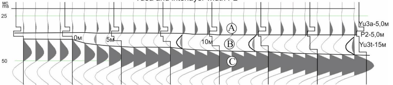
В. Изменение толщины межрезервуарной покрывки P2 при постоянной мощности пласта Ю3т и Ю3а
