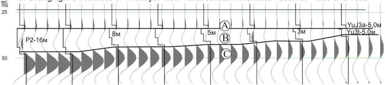
Г. Литолого-акустическая характеристика изучаемой части разреза
