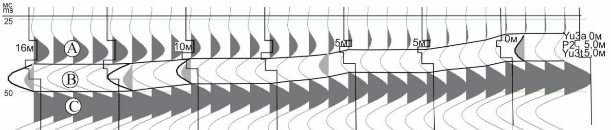
Б. Изменение толщины пласта Ю3т от 0 до 15 м при постоянной мощности пласта Ю3а и межрезервуарной покрывки P2
