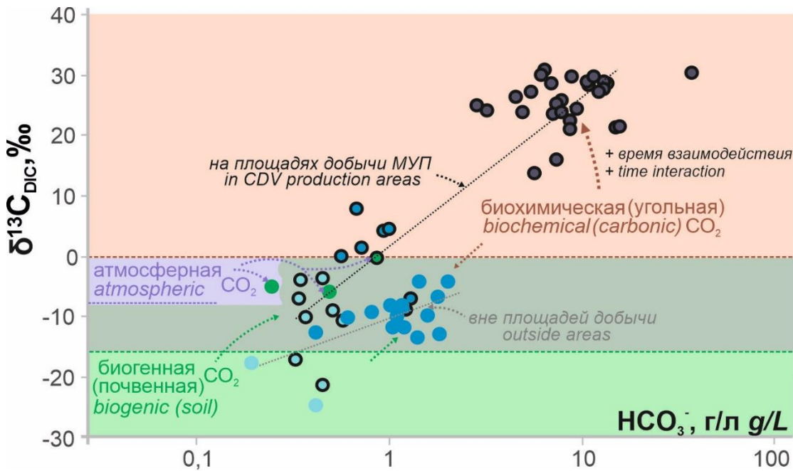
Рис. 5. Зависимости значений \delta^{13}\text{C}_{\text{DIC}} региона от концентрации гидрокарбонат иона. Жирным обведены точки с пробами на площадях добычи МУП
