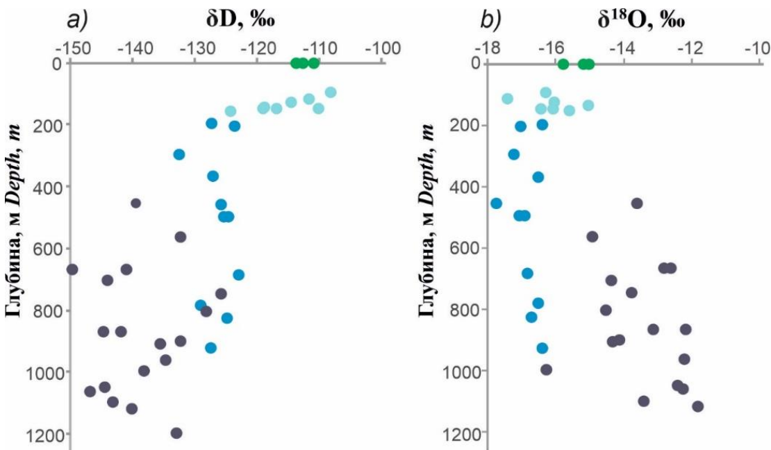
Рис. 3. Графики зависимости значений \delta\text{D} (a) и \delta^{18}\text{O} (b) вод от глубины залегания Fig. 3. Graphs of the dependence of \delta\text{D} (a) and \delta^{18}\text{O} (b) values of water on the depth of occurrence
