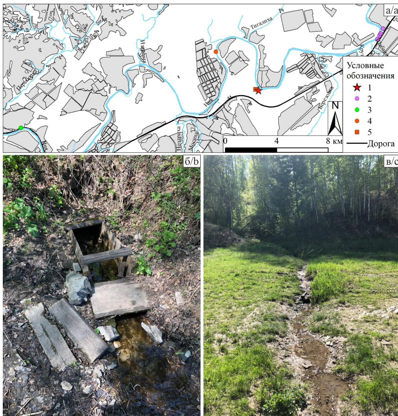
Рис. 1. Местоположение отбора проб (а), фотографии ключа Железнодорожный (б, в). Условные обозначения: 1 – Железнодорожный ключ; 2 – Инские источники; 3 – родник Новолуговой; 4 – родник Капустный; 5 – породы юргинской свиты
