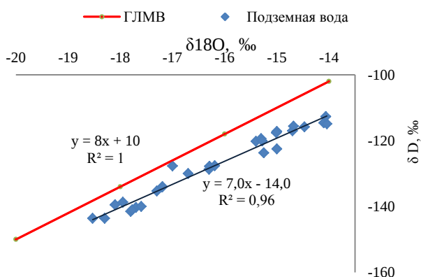
Рис. 2. Зависимость \delta^{18}\text{O} – \delta\text{D} в подземных водах Обь-Иртышского междуречья (ЛЛПВ) в 2022–2023 гг.
