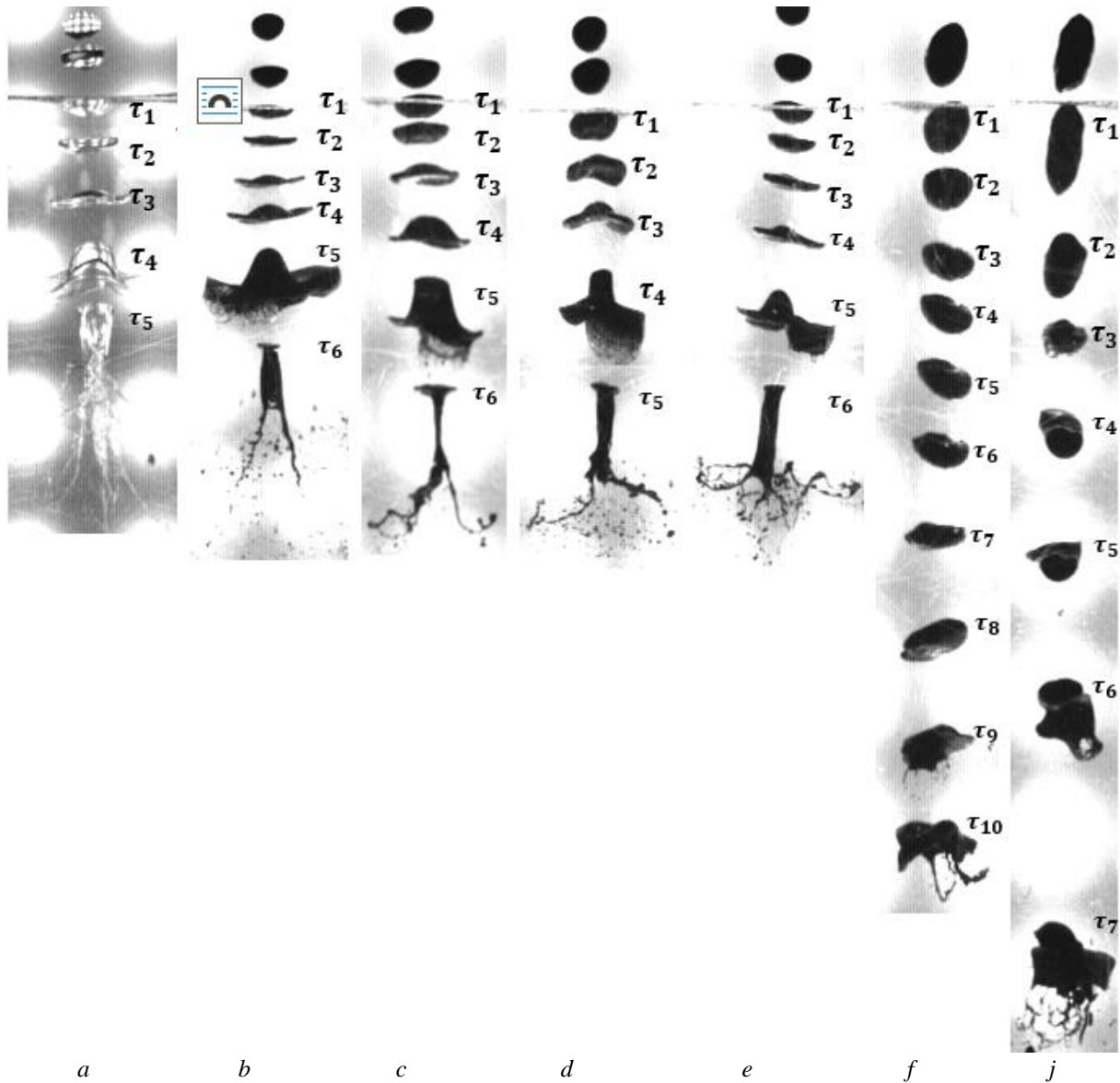
Рис. 2. Типичные кадры процесса диспергирования капель воды (a) и ВУТ (b–j). Соотношение в системе уголь/вода: a – 0/100; b – 10/90; c – 20/80; d – 30/70; e – 40/60; f – 50/50; j – 55/45
