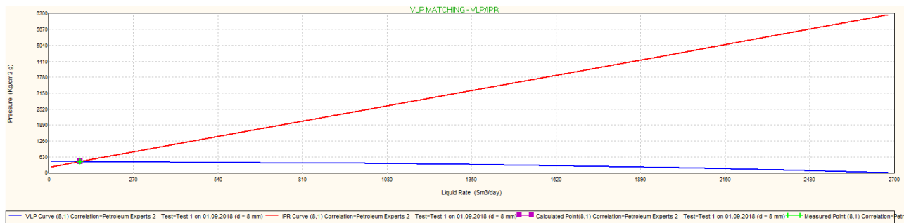
Рис. 8. Пересечение кривых VLP и IPR Fig. 8. Intersection of VLP and IPR curves
