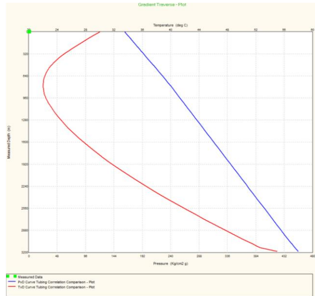
Рис. 7. График градиента давления Fig. 7. Pressure gradient plot
