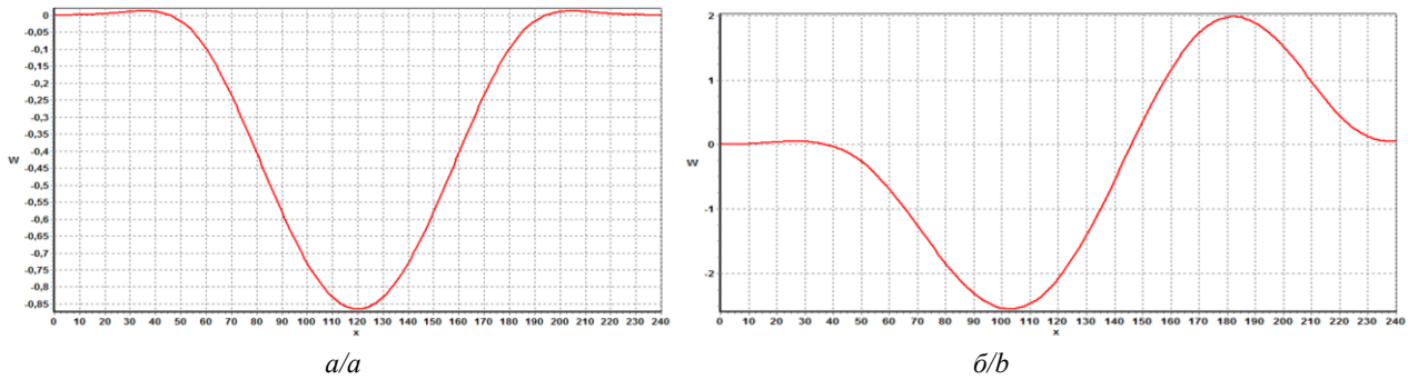
Fig. 5. Эпюры прогиба газопровода, балластированного 41 железобетонным утяжелителем марки 1-УБКм-1420-10 ( L=240 м, l=120 м, \gamma_{вод}=10,5 кН/м, Q_{yt}=32,70 кН), на болоте, указывающие на выпучивание трубы со стрелой прогиба, направленной вверх, параметры эксплуатации: а) p_0=7,5 МПа, \Delta t=47,0 °С; б) p_0=7,5 МПа, \Delta t=49,0 °С. Fig. 5. Diagrams of the deflection of the gas pipeline, ballasted with 41 reinforced concrete weights of the brand 1-UBKm-1420-10 ( L=240 m, l=120 m, \gamma_{вод}=10,5 кН/м, Q_{yt}=32,70 кН), in the swamp, indicating the bulging of the pipe with an upward deflection arrow, operating parameters: а) p_0=7.5 МПа, \Delta t=47.0^\circ\text{C} ; б) p_0=7.5 МПа, \Delta t=49.0^\circ\text{C}
