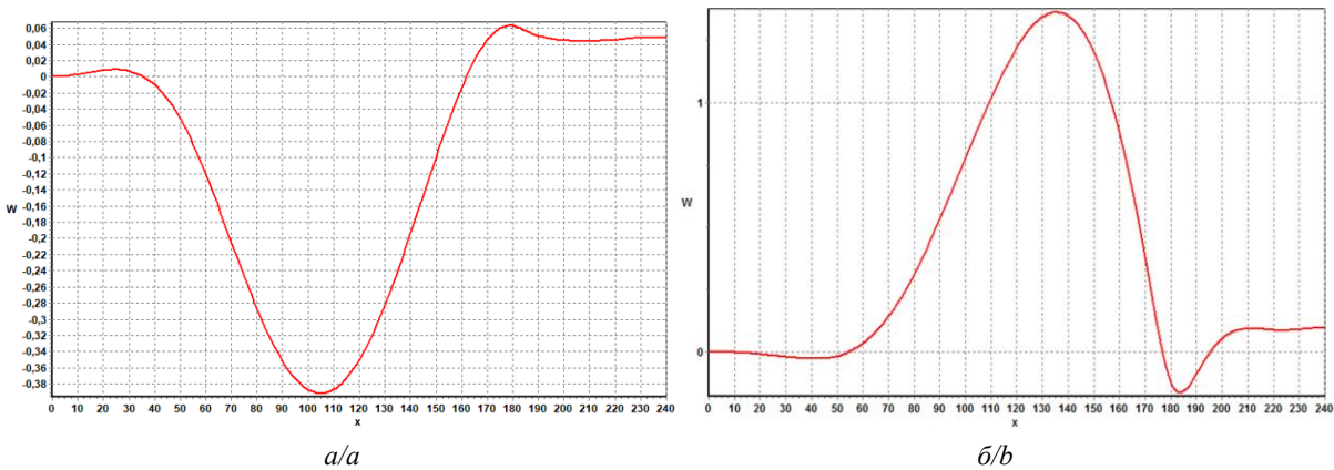
Fig. 6. Эпюры прогиба газопровода, балластированного 41 железобетонным утяжелителем марки 1-УБКм-1420-10 ( L=240 м, l=120 м, \gamma_{вод}=10,5 кН/м, Q_{yt}=32,70 кН), на болоте, при неравномерном неодинаковом ослаблении грунта в подземных частях, параметры эксплуатации: а) p_0=7,5 МПа, \Delta t=32,50 °С; б) p_0=7,5 МПа, \Delta t=33,40 °С. Fig. 6. Diagrams of the deflection of the gas pipeline, ballasted with 41 reinforced concrete weights of grade 1-UBKm-1420-10 ( L=240 m, l=120 m, \gamma_{вод}=10,5 кН/м, Q_{yt}=32,70 кН), in the swamp with uneven weakening of the soil in the underground parts, operating parameters: а) p_0=7.5 МПа, \Delta t=32.50^\circ\text{C} ; б) p_0=7.5 МПа, \Delta t=33.40^\circ\text{C}
