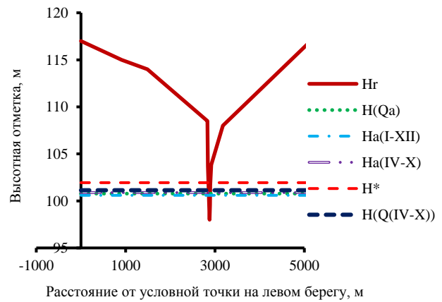
Рис. 3. Профиль долины р. Иксы у с. Плотниково и средние уровни воды, рассчитанные различными способами (табл. 1); Hr – высотная отметка поверхности водосбора и дна реки; остальные обозначения – в табл. 1
