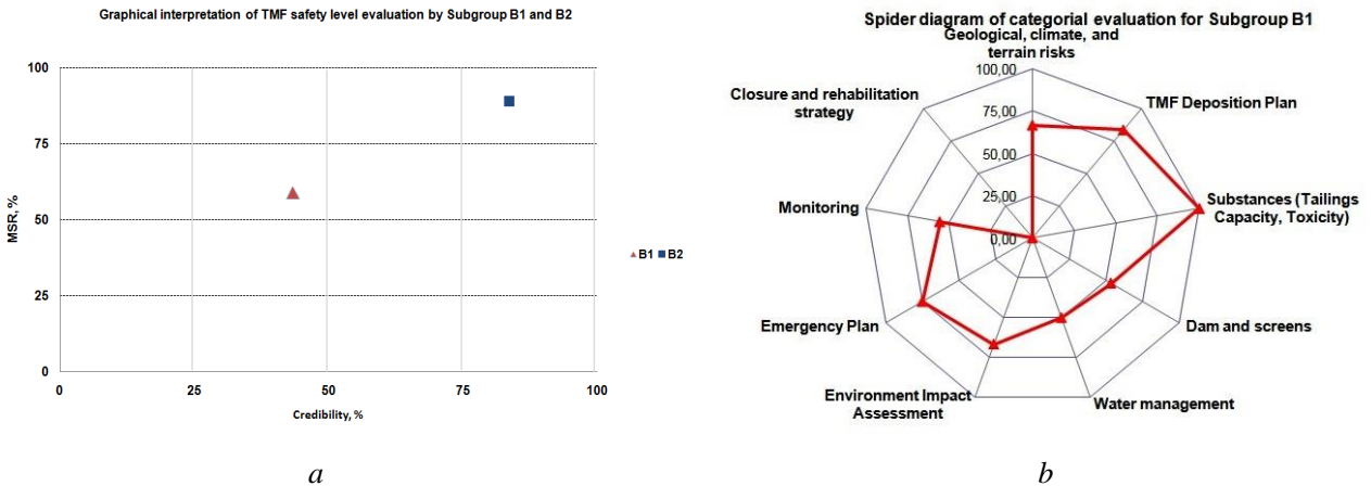
Fig. 2. Safety evaluation results for the main dam: a) overall evaluation; b) categorial evaluation for visual check Рис. 2. Результаты оценки безопасности главной плотины: а) общая оценка; б) категориальная оценка визуального осмотра
