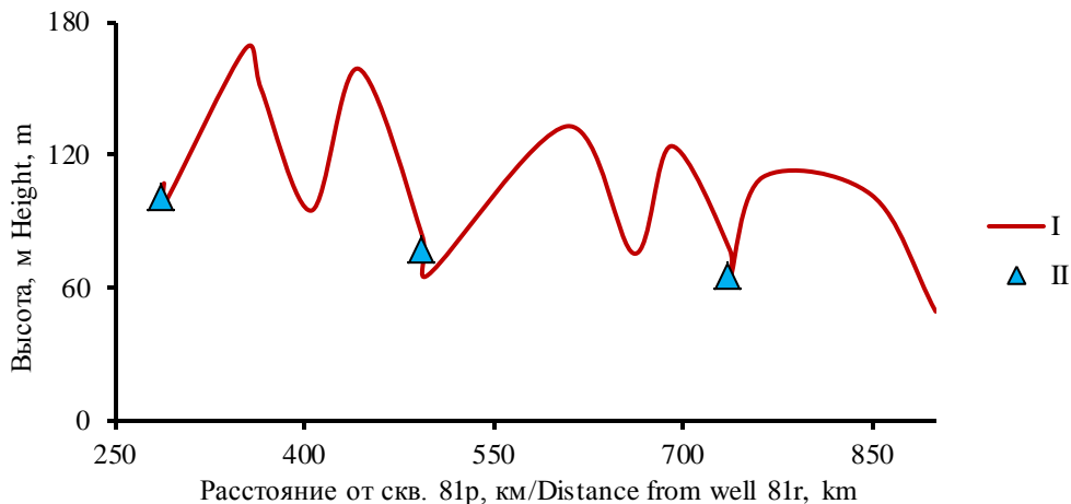
Рис. 6. Схематичный профиль поверхности (I, включая уровни речных вод) и среднемноголетние уровни подземных вод (II: 81р, 113р, 156р) на участке от с. Зырянское до уреза воды р. Вах у с. Ларьяк
