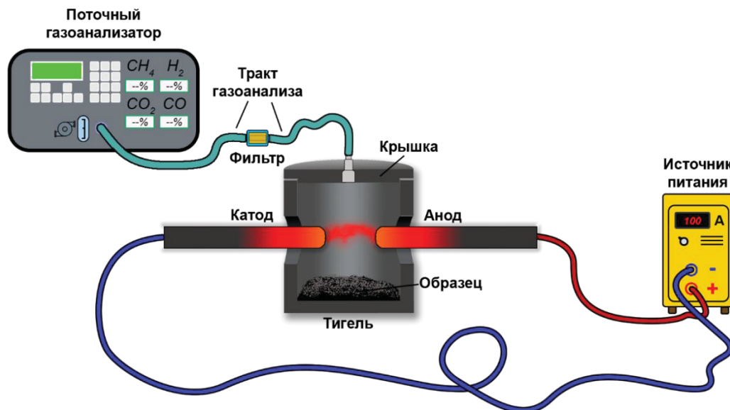
Рис. 1. Безвакуумный электродуговой реактор постоянного тока с горизонтальным расположением электродов Fig. 1. Vacuumless DC electric arc reactor with horizontal electrode arrangement
