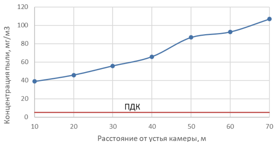
Рис. 4. Результаты измерения массовой концентрации пыли в очистной выработке
