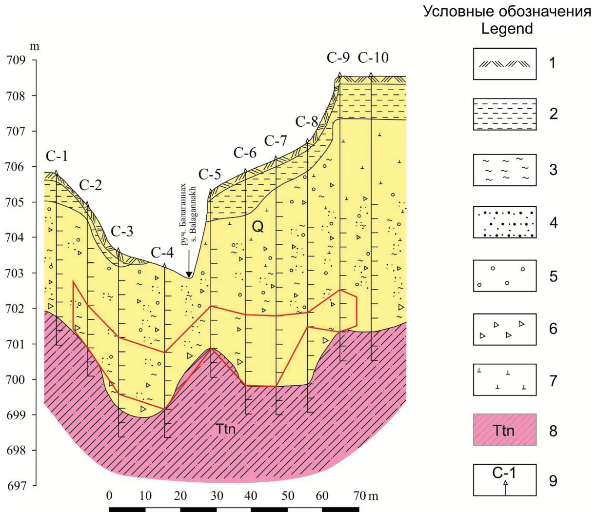
Рис. 2. Разрез по разведочной линии № 126. Четвертичные отложения (Q) 1–6: 1 – почвенно-растительный слой, 2 – ил, 3 – глина, 4 – песок, гравий, 5 – галька, валуны, 6 – щебень, древесная; 7 – лед; 8 – Тонорская свита (Ttn) – алевропесчаники; 9 – скважина и ее наименование; красная линия – контур рудного тела. Вертикальный масштаб 1:100, горизонтальный – 1:1000
