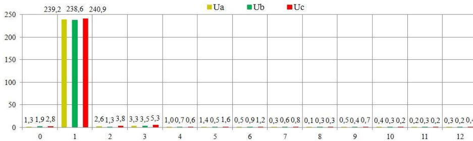
Рис. 4. Гармонический спектр генерируемых напряжений в режиме холостого хода Fig. 4. Harmonic spectrum of produced voltages at no-load mode
