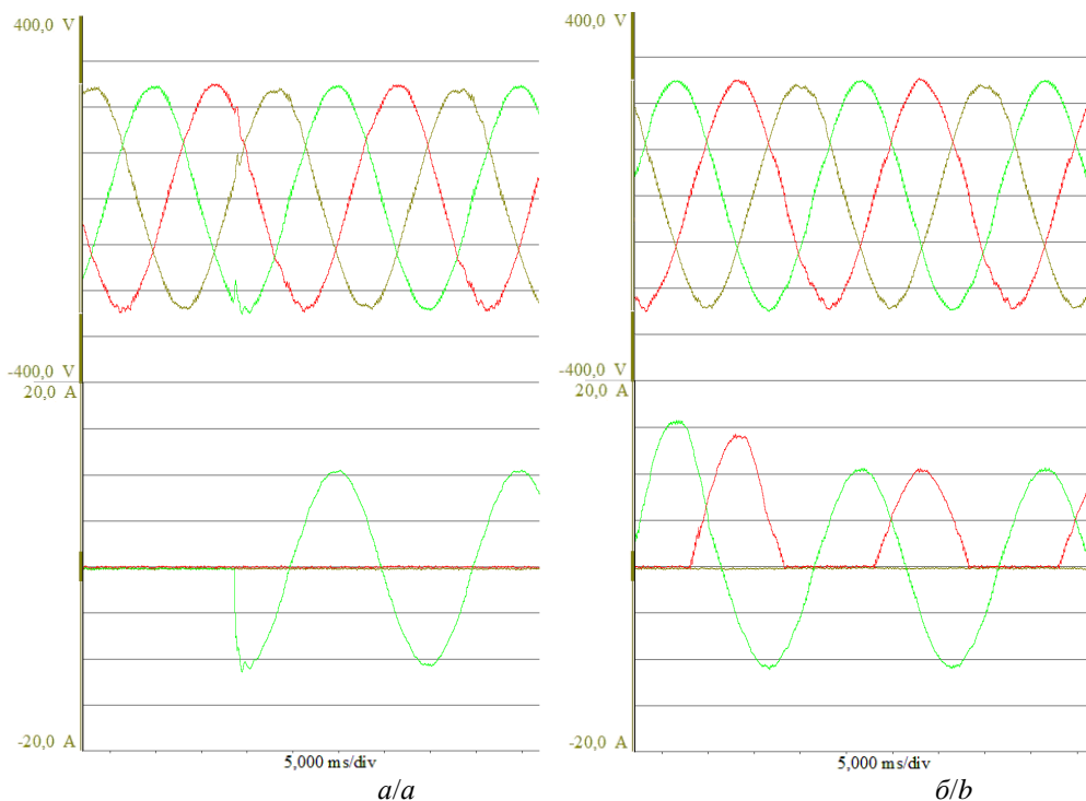
Рис. 5. Трехфазные напряжения и токи на стороне потребителя при скачкообразном изменении однофазной (а) и двухфазной (б) нагрузки Fig. 5. Load three-phase voltages and currents under step change of single-phase (a), two-phase (b) loads
