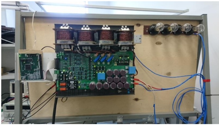
Рис. 3. Внешний вид экспериментальной установки Fig. 3. Photograph of experimental platform
