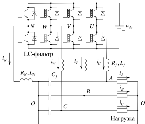
Рис. 1. Упрощенная функциональная схема трехфазной системы электроснабжения на базе четырехстоечного мостового инвертора
