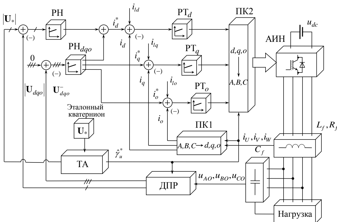
Рис. 2. Система управления четырехстоечным преобразователем в кватернионном базисе Fig. 2. Control system of the four-leg VSI in quaternion domain
