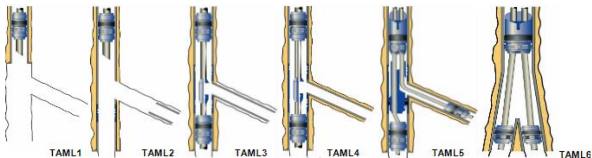
Рис. 2. Классификация уровней сложности многоствольных скважин TAML
