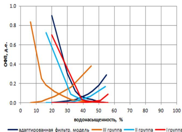
Рис. 2. Адаптированная фильтрационная модель нефти, воды и лабораторные кривые ОФП, средние по группам образцов породы пласта ВЧ. Группы образцов по гранулометрической фракции: I – песчаник среднелкозернистый, хорошо отсортированный, однородный; II – разнотзернистый песчаник, слабогравелистый, с незначительным засолением; III – грубозернистый, плохосортированный песчаник, гравелистый, с повышенной степенью засоления либо гравелит разнообломочный, песчанистый
