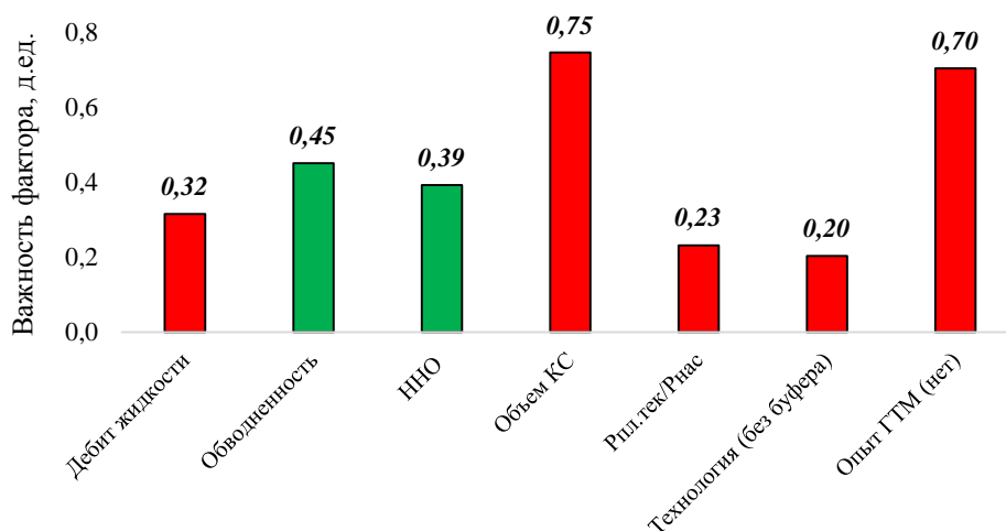
Рис. 6. Относительное влияние факторов, вошедших в итоговую модель классификации
