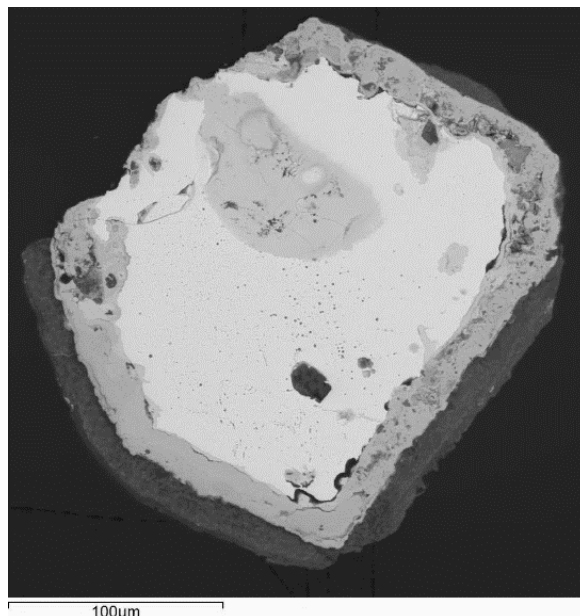
Рис. 7. Зерно торита с частично кристаллогранной формой, периферическая зона (тёмно-серая) сложена ториянитом
