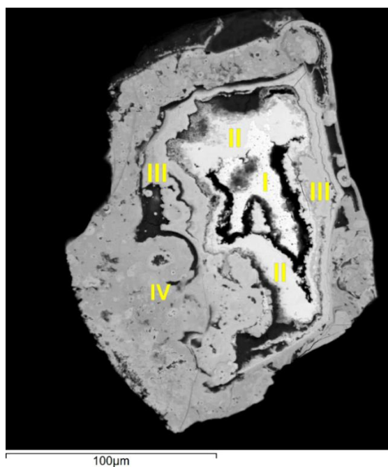
Рис. 8. Зерно торита
