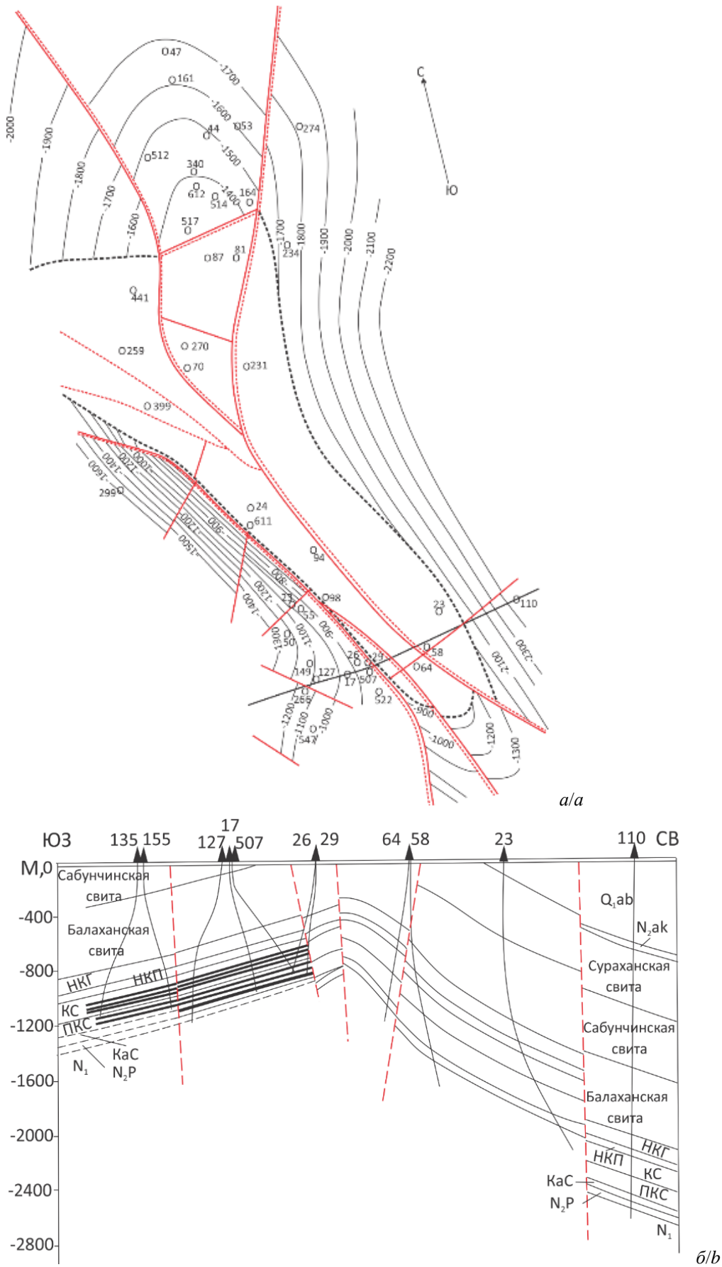
Рис. 2. Месторождение Дарвин кюпеси: а) структурная карта по кровли ПКС; б) геологический профиль по линии I-I Fig. 2. Deposit Darwin kypesi: a) structural map for the roof of the PKS; b) geological profile along the line I-I
