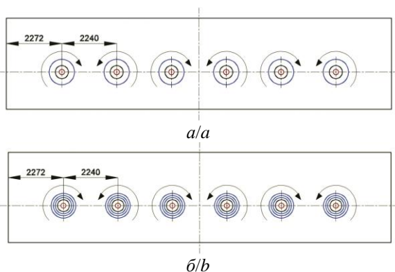
Рис. 2. Схема размещения горелок с направлением вращения: а) проектных горелок; б) малоэмиссионных горелок Fig. 2. Scheme of burners with a marked swirl direction: a) design burners; b) low emission burners
