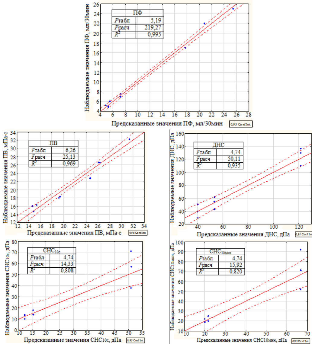
Рис. 1. Графики наблюдаемых и предсказанных по уравнениям регрессий значений показателя фильтрации (ПФ) и реологических параметров (ПВ, ДНС, СНС 10с и СНС 10мин ) при доверительной вероятности p=0,95 (пунктирная линия – доверительный интервал)
