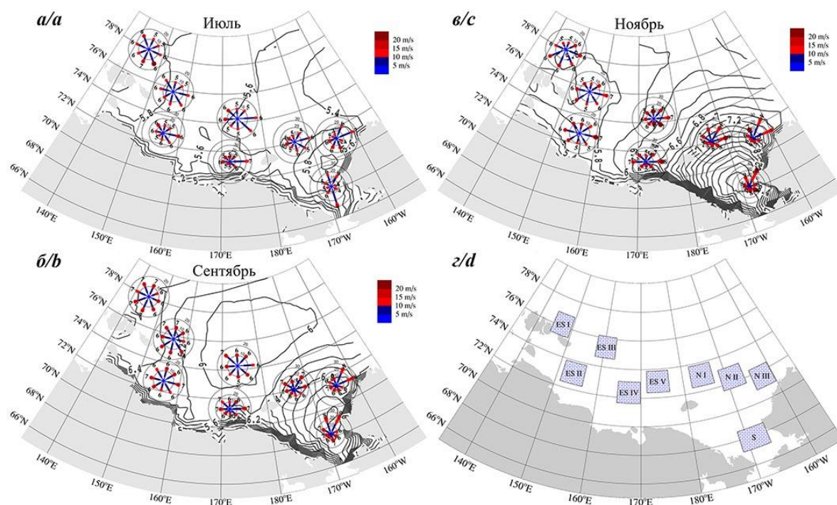
Рис. 1. Средняя скорость ветра для Чукотского и Восточно-Сибирского морей и розы ветров в июле (а), сентябре (б) и ноябре (в). Изоханы проведены через 0,2 м/с для скоростей ветра более 5 м/с и через 0,5 м/с для скоростей менее 5 м/с; на лучах роз ветров указана средняя скорость данного направления ветра. (г) Районы Чукотского и Восточно-Сибирского морей
