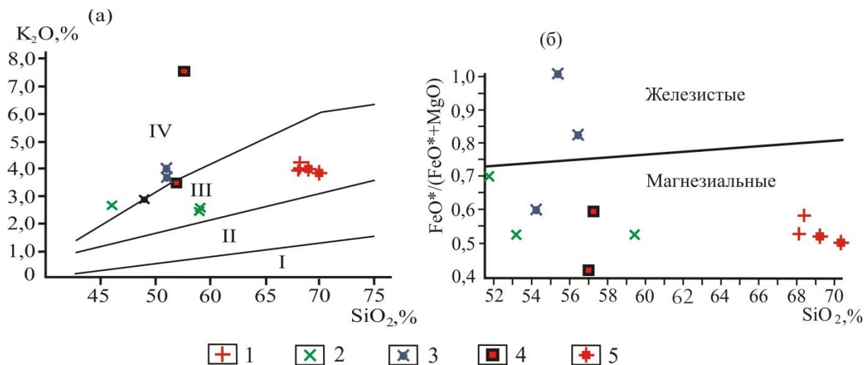
Рис. 4. Диаграммы K_2O-SiO_2 (а), FeO^*/(FeO^*+MgO)-SiO_2 (б) для интрузий Александровского месторождения. Бичурский комплекс ( P_2 ): 1 – гранитоиды, 2 – кварцевые диориты; Амуджикано-Шахтаминский комплекс (дайки): 3 – микродиориты, 4 – гранит-порфиры, 5 – гранитоиды. а) Поля интрузивных серий на диаграмме: IV – шошонитовая, III – высококальциевая известково-щелочная, II – среднекальциевая известково-щелочная, I – островодужная; б) Поля железистых и магнезиальных гранитоидов [11]
