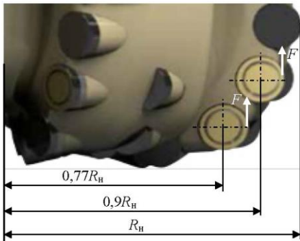
Рис. 4. Торцевая часть долота с резами ONYX
