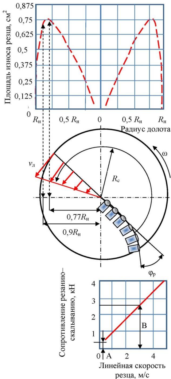
Рис. 3. Схема установки резов на торце долота с учетом скоростей резания-скалывания породы и интенсивности изнашивания резов
