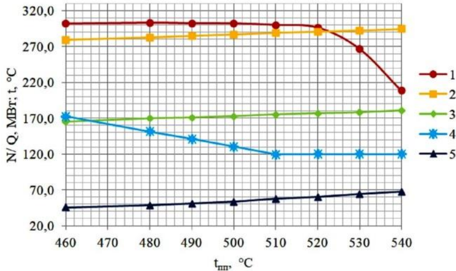
Рис. 4. Зависимость показателей работы ПГУ в теплофикационном режиме от температуры промежуточного перегрева пара: 1 – Q_m ; 2 – N_e^{ncy} ; 3 – N_e^{nm} ; 4 – t_{yx} ; 5 – Q_k
