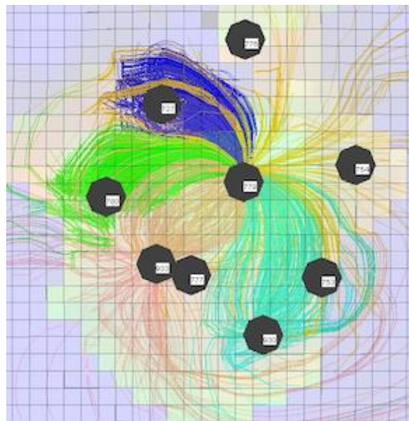
Рис. 2. Направления фильтрационных потоков на участке залежи
