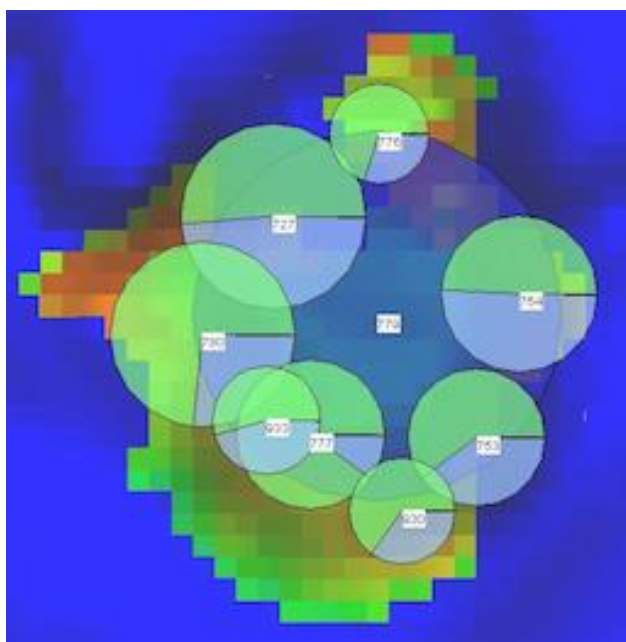
Рис. 1. Карта накопленных отборов и закачки на поднятии Fig. 1. Map of cumulative oil production and water injection
